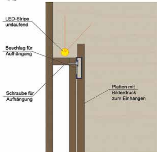
Detail-Schnitt durch Bilder M 1:2
